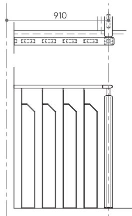
●吹抜け部手摺 1P 間口 (910) [階段手摺~壁納め]
