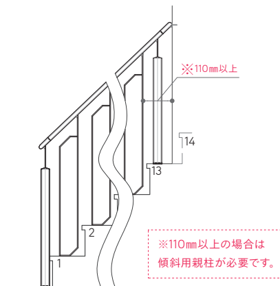
●階段手摺 直 14 段上りきり [壁納め]
