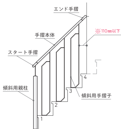
●階段手摺 上り始め直 4 段上りきり [壁納め]
